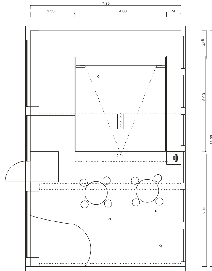
Grundriss
